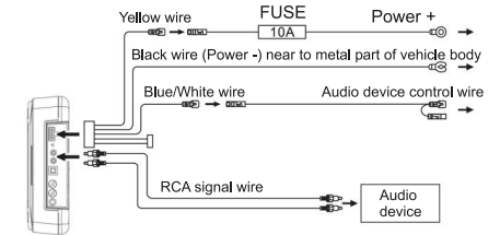
Anschlussdiagramm 2 (Chinch-Eingang)
