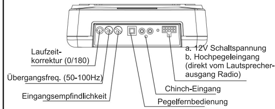
Funktionskontrolldiagramm
